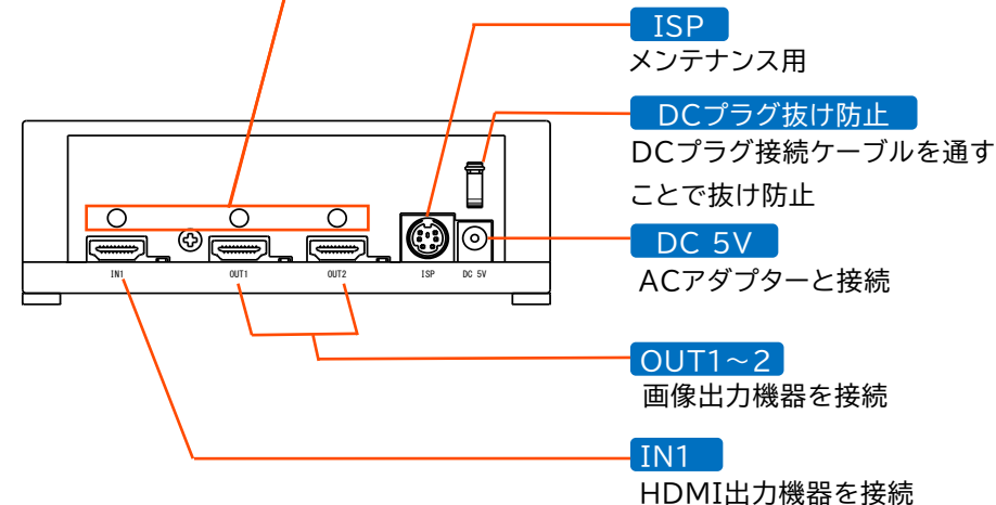
LSP-HD12 背面図
