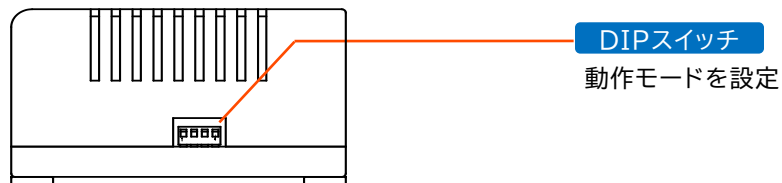
LSP-HD12 側面図
